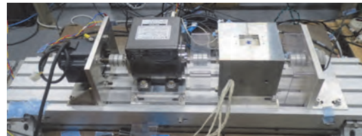
コア損を計測するモータシミュレータ
