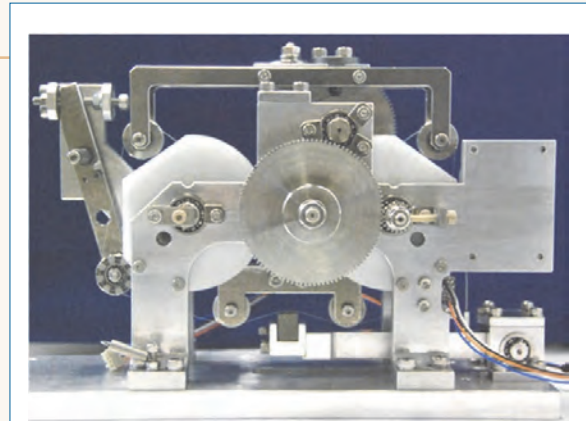
ワイヤソー切断装置の外観
